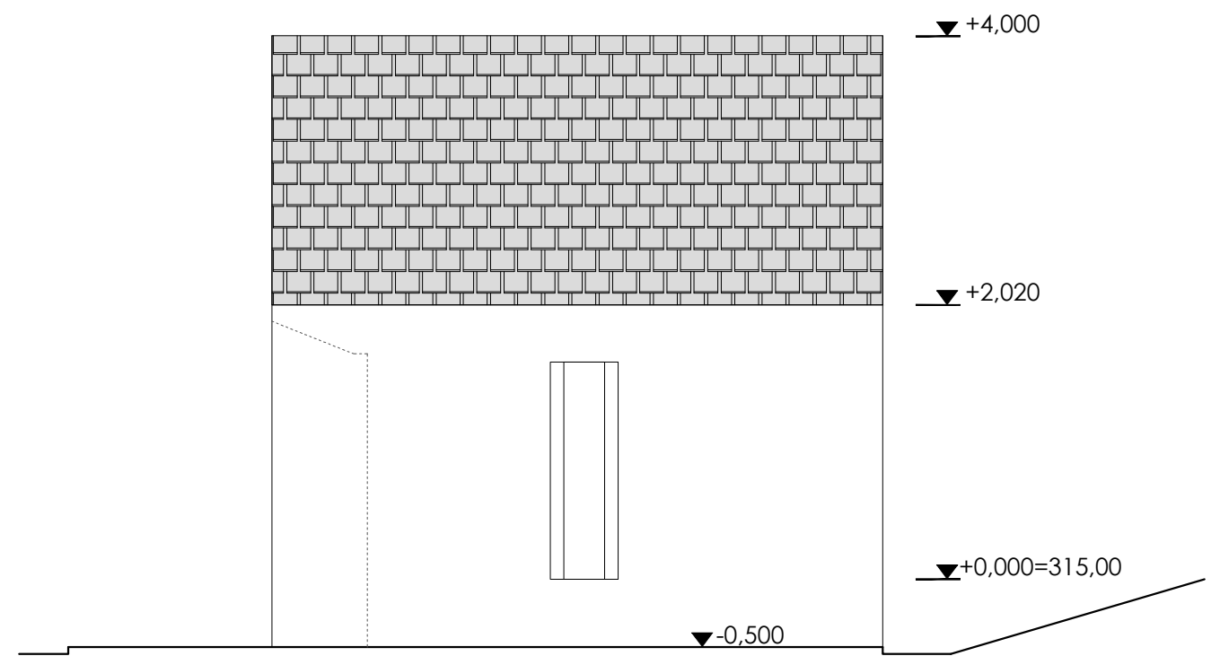
POHLED JIŽNÍ 1:50
