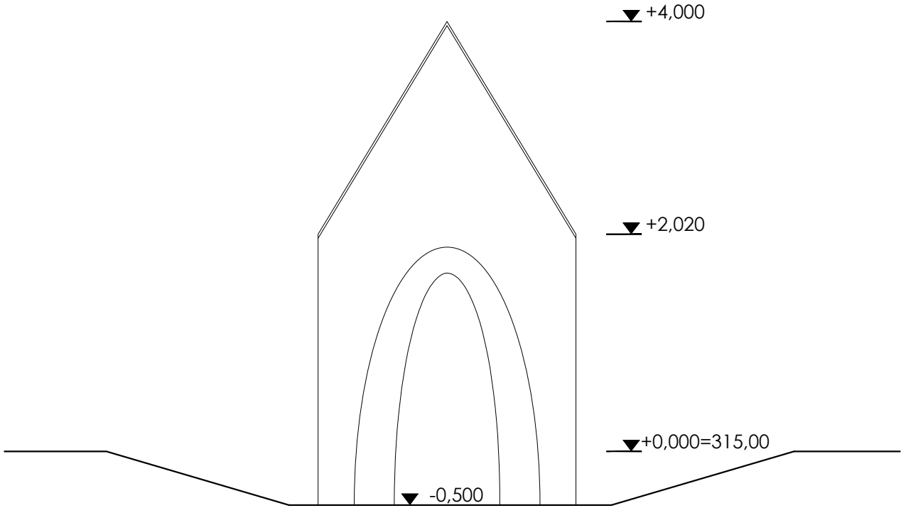
POHLED ZÁPADNÍ 1:50
