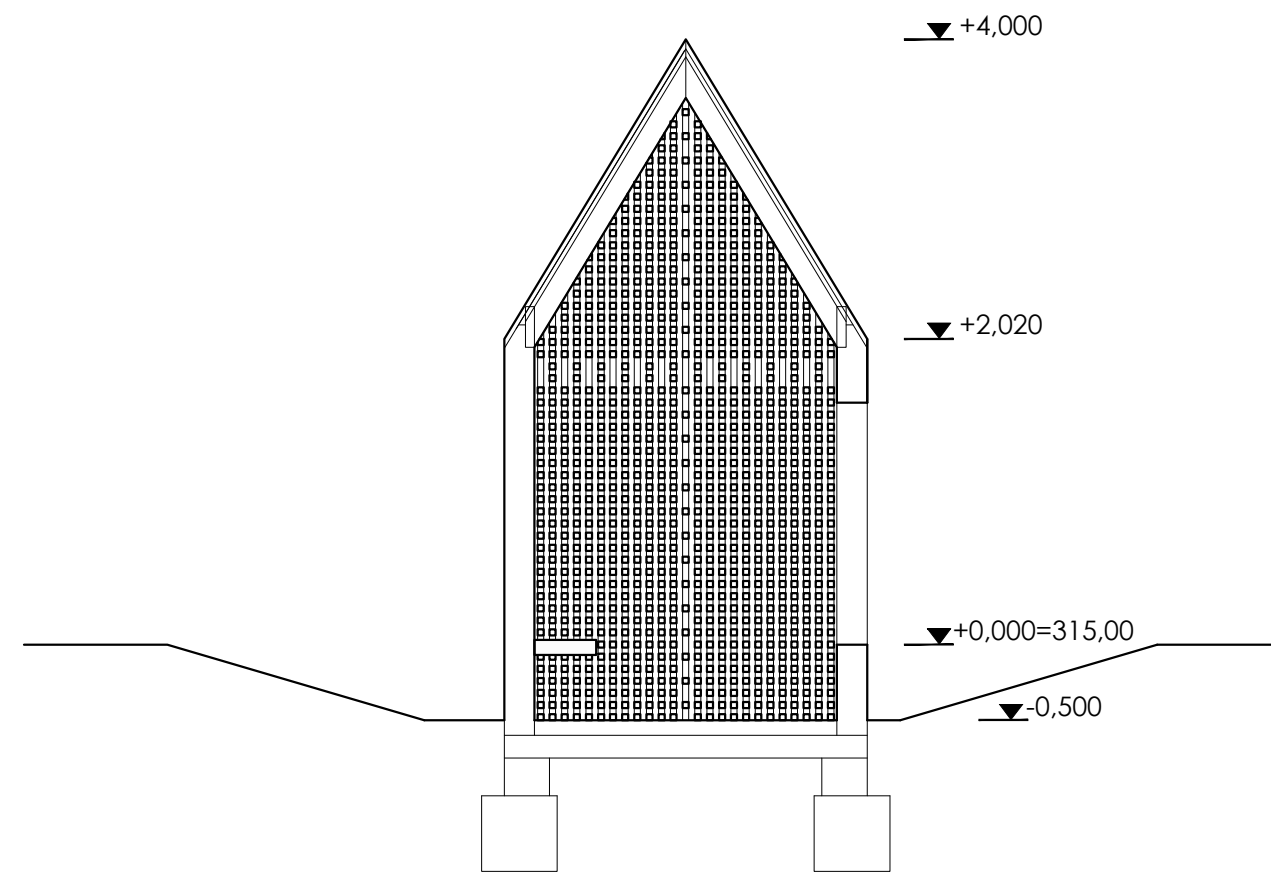
ŘEZ A-A' 1:50
