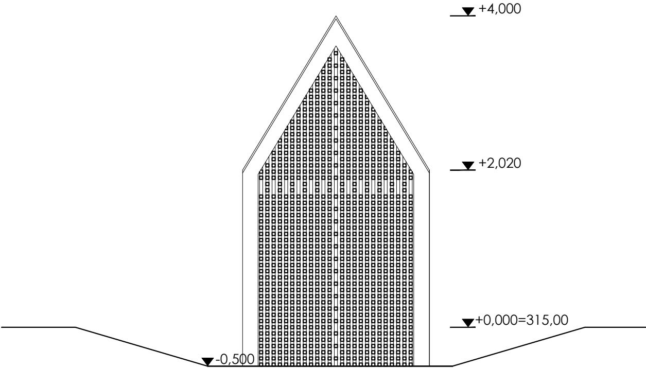
POHLED VÝCHODNÍ 1:50
